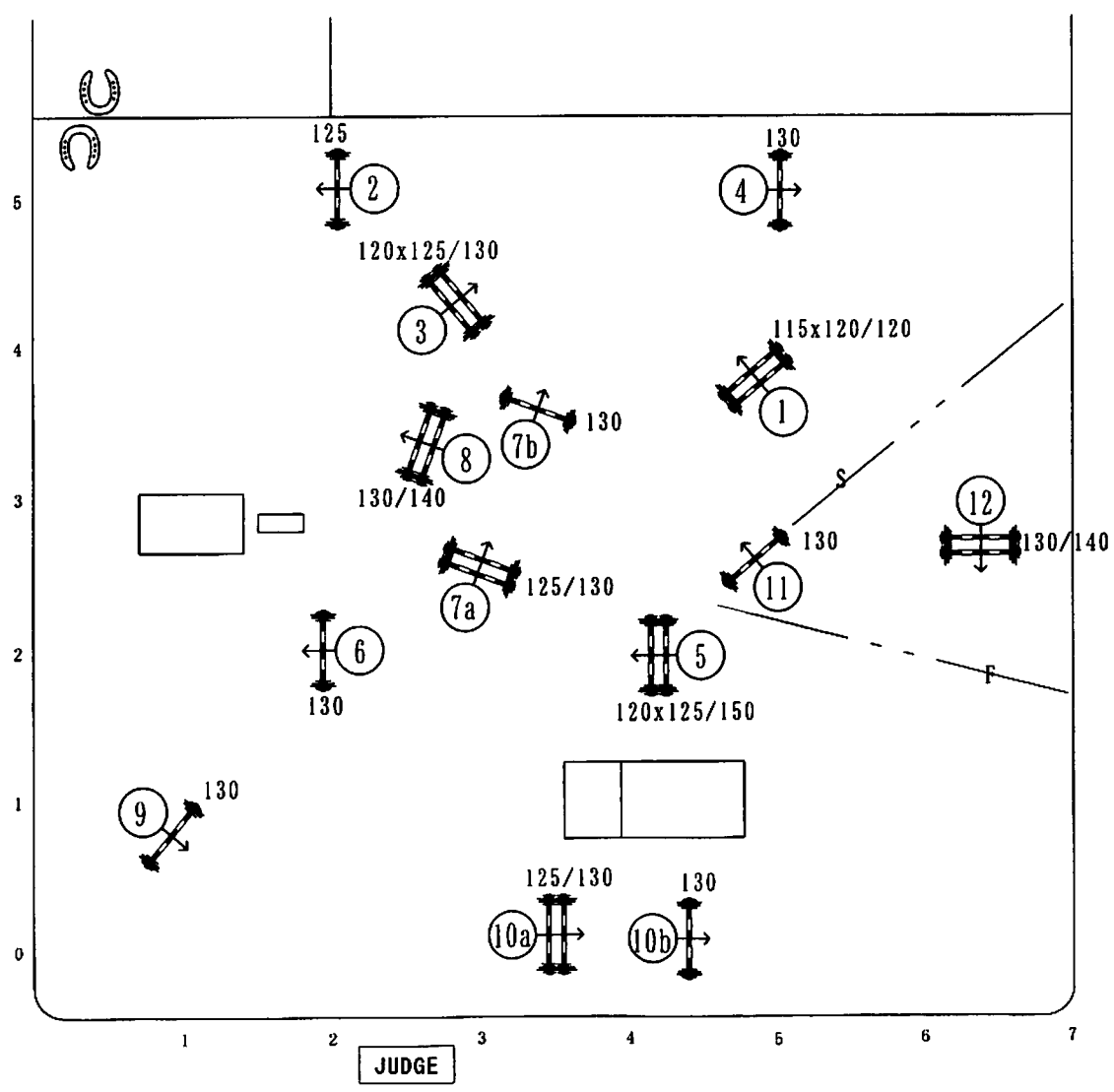
[経路図 1/500]
