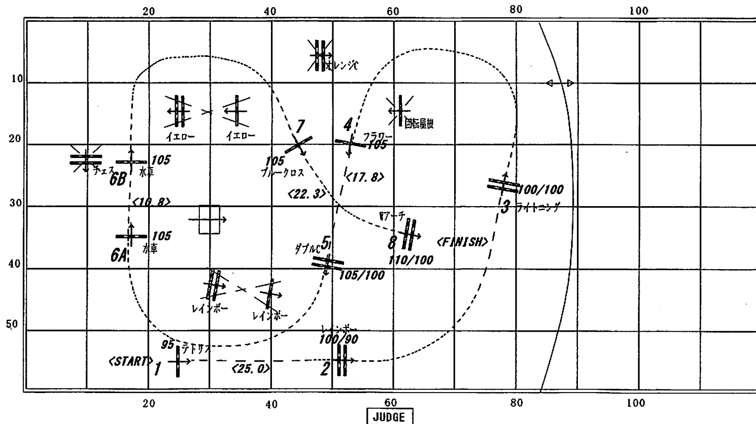
[経路図 1/ 500]
